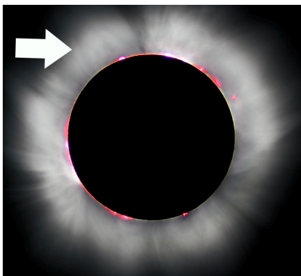
corona
