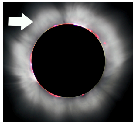
corona
